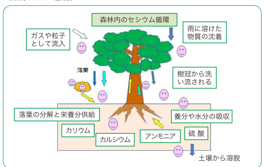
■森林内のセシウム循環図
